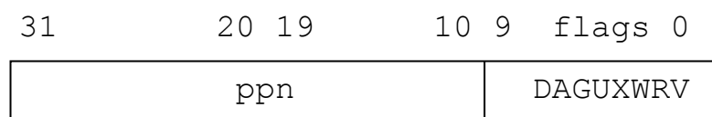
Figura 9: Formato de una page table entry (pte).
