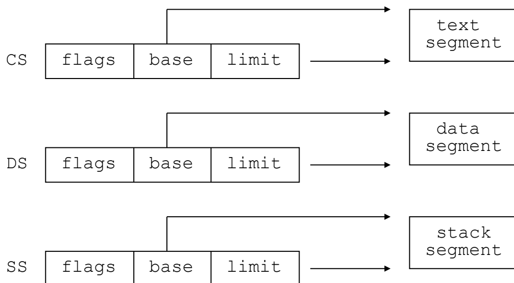
Figura 3: Registros de segmentos.
